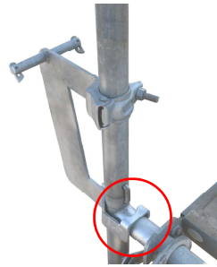
AA-TKを使用すると横架材で位置合わせができます
