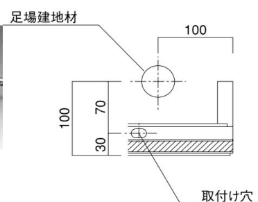
コーナーパネルクランプ BP-CK 0.50 kg コーナー部
