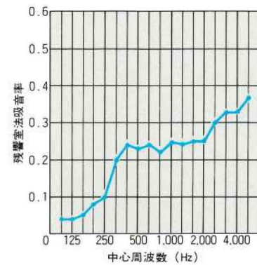
● 残響室法吸音性能試験結果
