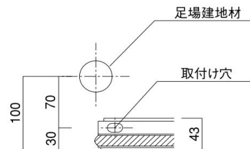
兼用パネルクランプ BP-42K 0.48 kg 直線部
