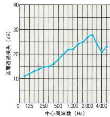
● 遮音性能試験結果
