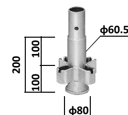
ポケット金具 TS-P2 3.4 kg
