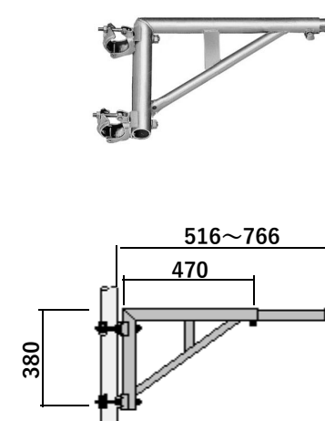
伸縮ブラケット TS-500C 5.3 kg
