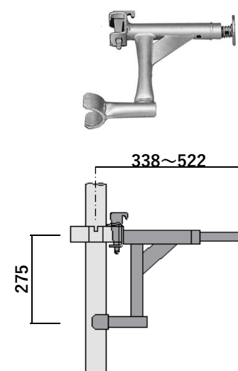
方杖付スライド腕木 TS-500 3.94 kg
