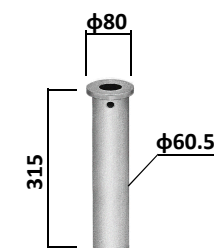
ロングカラー材 TS-HCL 2.1 kg
