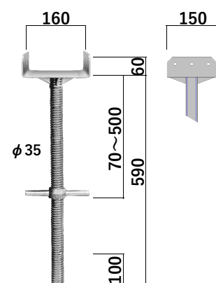
ロング大引受ジャッキ A-752HS 溶融亜鉛メッキ 6.5 kg
