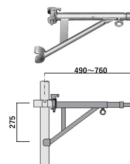
方杖付スライド腕木 TS-750 4.61 kg
