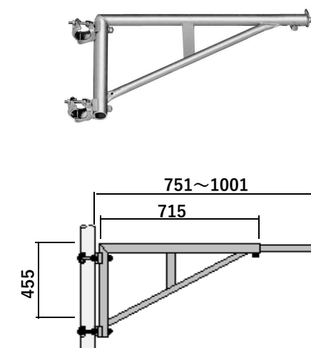
伸縮ブラケット TS-750C 6.5 kg
