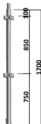
建地材 TS-P17 11.6 kg
