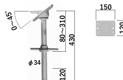
ピポットジャッキ A-14P 溶融亜鉛メッキ 4.1 kg
